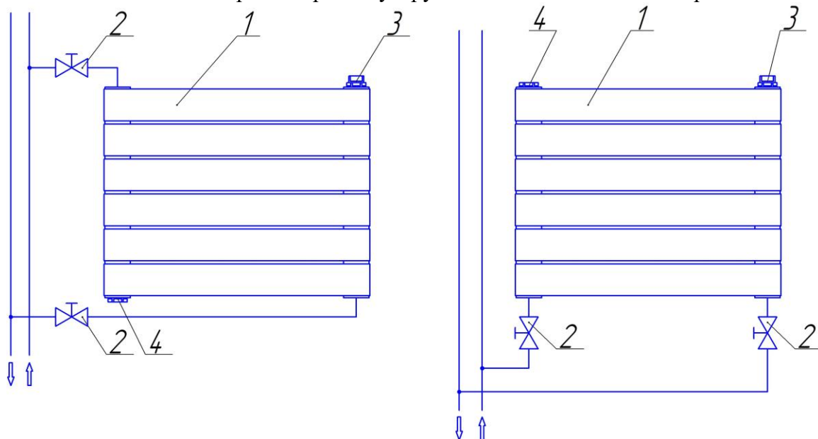
Рис. 3 1. Радиатор. 2. Вентиль (кран). 3. Кран Маевского-воздухоотводчик. 4. Пробка глухая.
